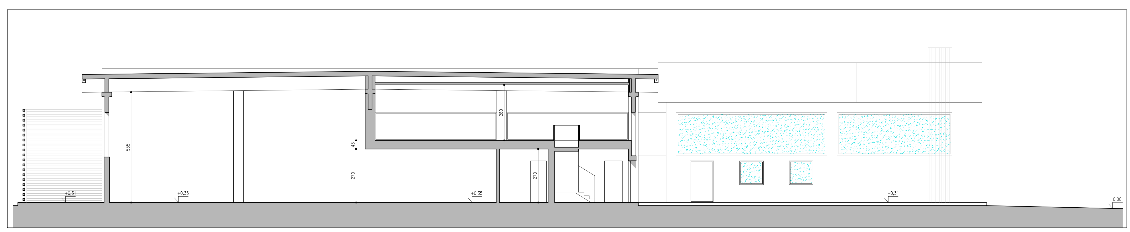
SEZIONE A-A
